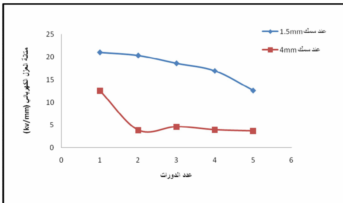
الشكل (4) يوضح متانة العزل مع عدد الدورات لآتمودج (96% Polyester +4% Alumina) لمعدل صعود الفولتية (5 kV/sec).
