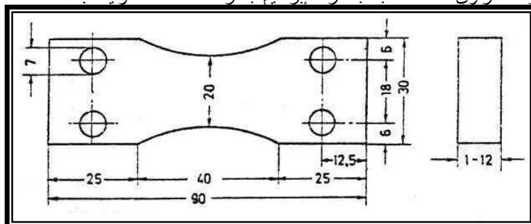
شكل (1-1) نموذج اختبار الإعياء بالأبعاد في mm .
