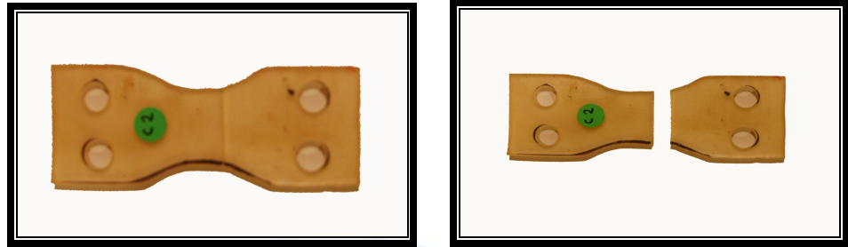
الصور الفوتوغرافية لمترابكات الايبوكسي بعد اختبار الكلال.
