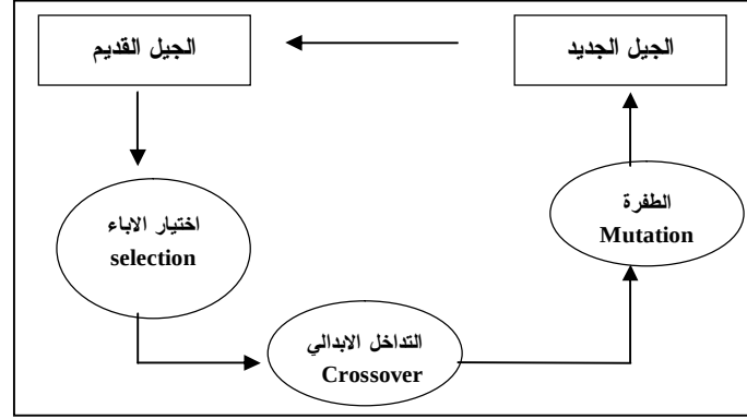
الشكل (1) يوضح دورة حياة الخوارزمية الجينية
