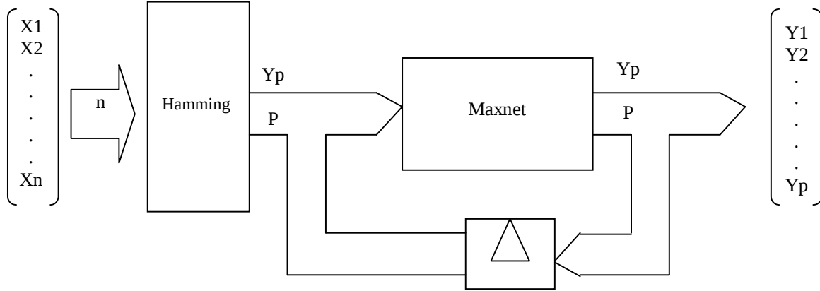
الشكل ( 3 ) المخطط الصندوقي لشبكة Hamming & Maxnet
