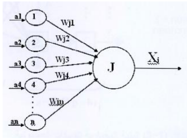
الشكل ( 2 ) مكونات العصبون
