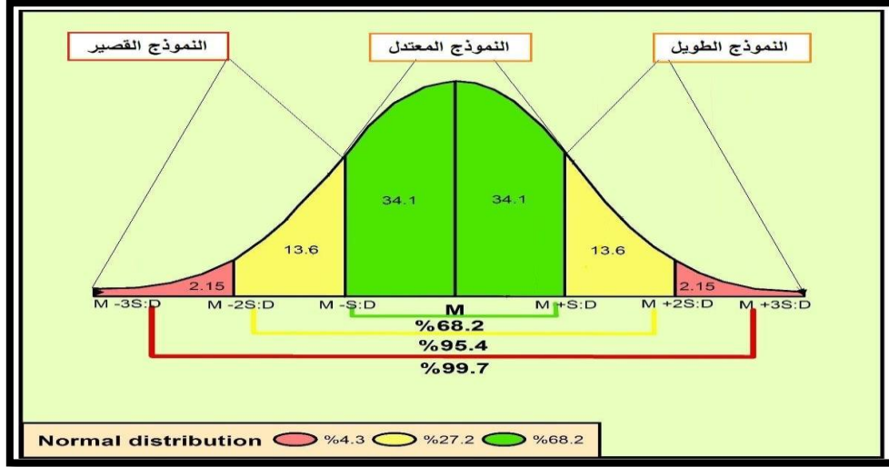
الشكل (١) التوزيع الطبيعي Normal Distribution للبيانات المعلمية
