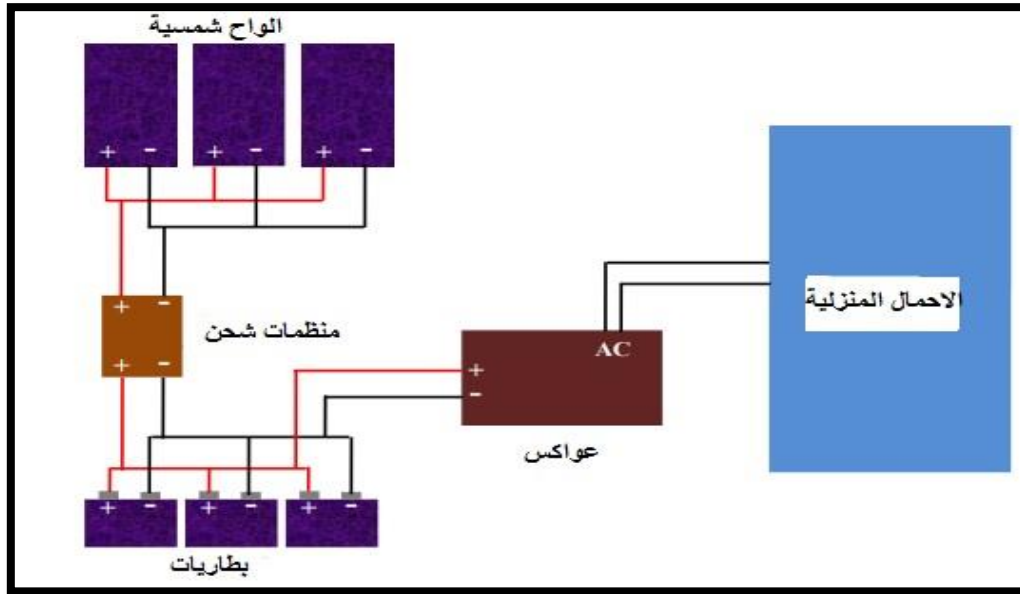
الشكل (٢) رسم تخطيطي لمنظومة الألواح المستقلة (of-grid)
