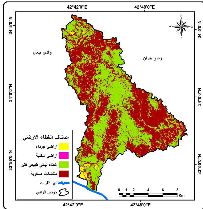
خريطة (٦) أصناف الغطاء الأرضي لحوض وادي العبيدي
