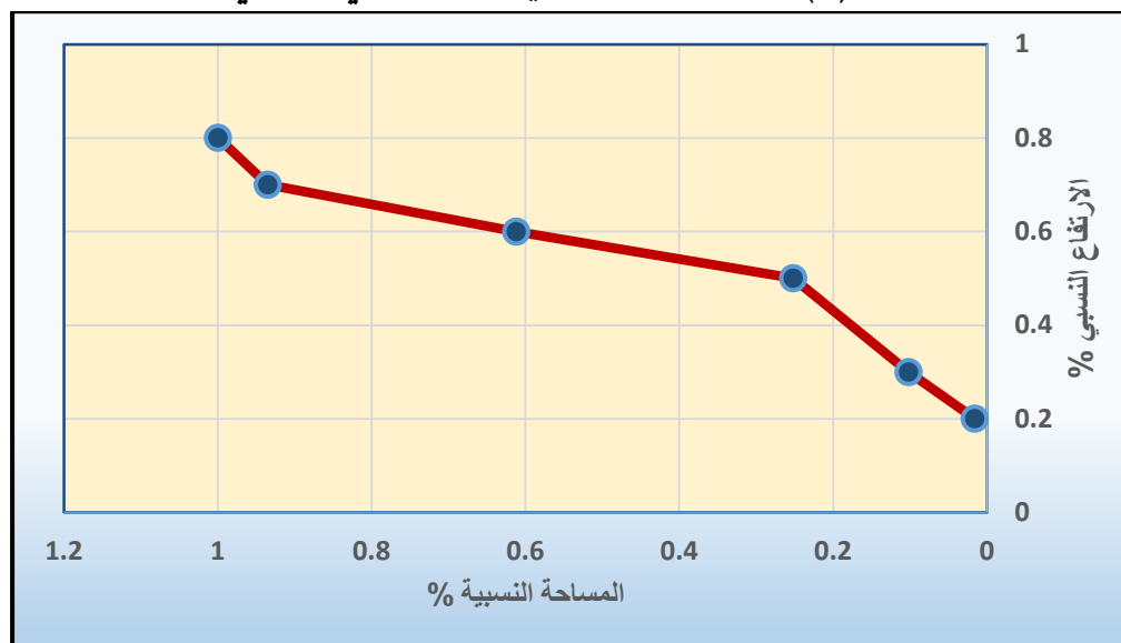
شكل (١) المنحنى الهيسومتري لحوض وادي العبيدي
