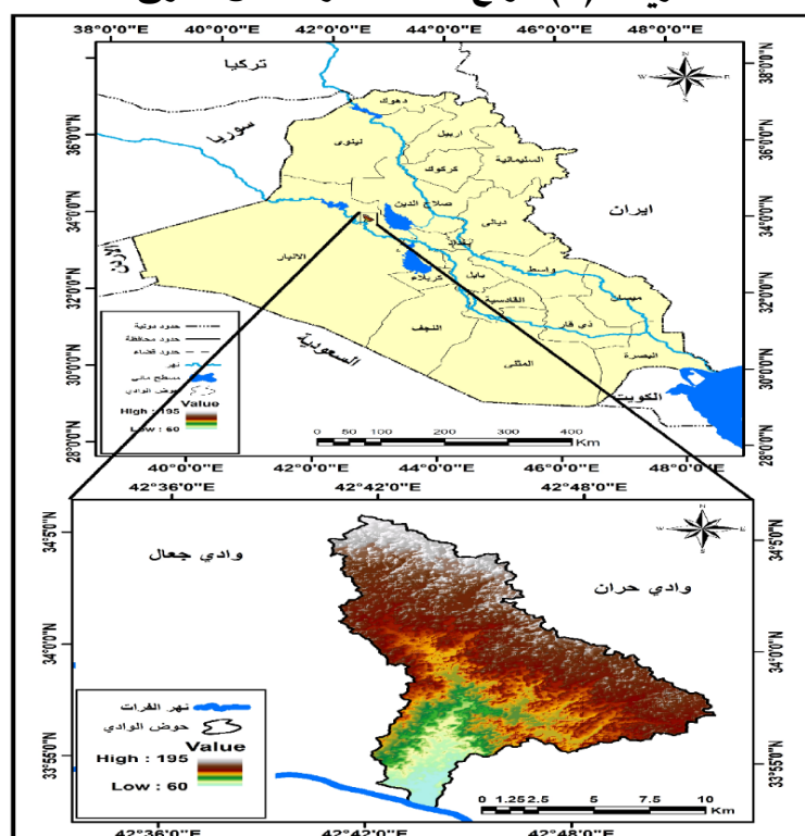
خريطة (١) موقع منطقة الدراسة من العراق
