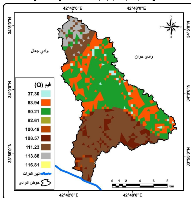
خريطة (١٠) قيم (Q) لحوض وادي العبيدي
