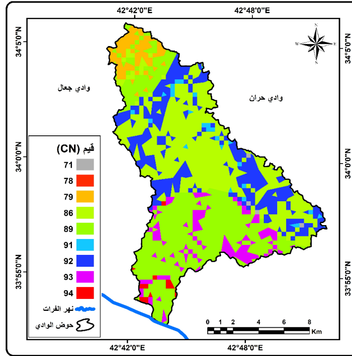
خريطة (٧) توزيع قيم (CN) لحوض وادي العبيدي
