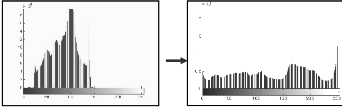
المدرج التكراري لصورة الموزائيك بعد عملية بسط التباين الخطي المدرج التكراري قبل وبعد عملية البسط الخطي للتباين الشكل (4): المدرج التكراري قبل وبعد عملية البسط الخطي للتباين
