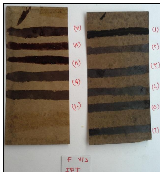
صورة رقم (٤) حبر بيروجالات الحديد الباهت قبل وبعد الانعاش بمحاليل الدراسة العشرة في شكل خطوط
