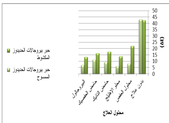
جدول رقم (١٩) ونمطه الإحصائي لقيم ΔE لألوان ترميم بيروجالات الحديدك المكشوط
