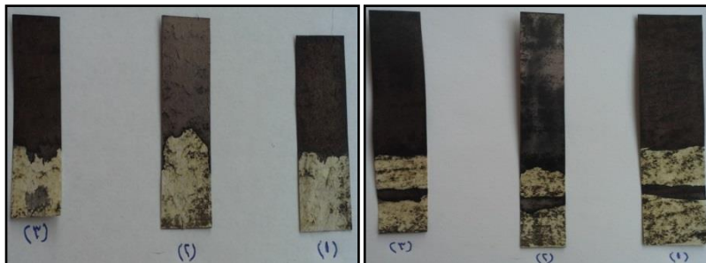
صورة رقم (١٣) حبر تانات الحديد المكشوط والممسوح بعد ترميمه وإنعاشه بمحاليل حامض العفصيك، التانيك والبيروجالول المثارة بالموجات فوق الصوتية (مثال)
