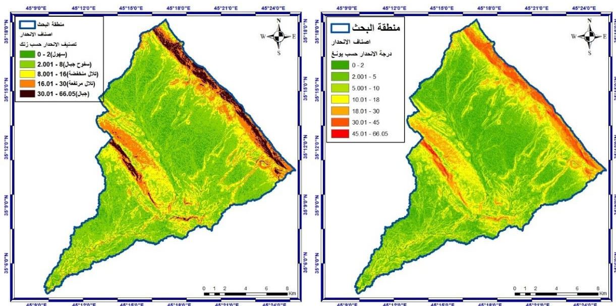
خريطة (٥) تصنيف الانحدار حسب يونغ.
