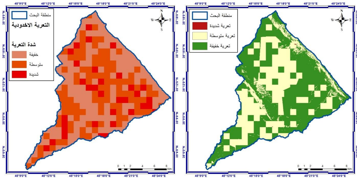
خريطة (١٢) تطابق خرائط أنواع التعرية.
