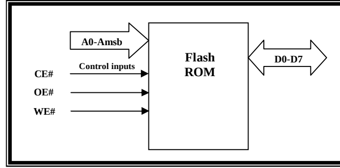
الشكل (1) : المخطط الصندوقي لذاكرة (Flash ROM)
