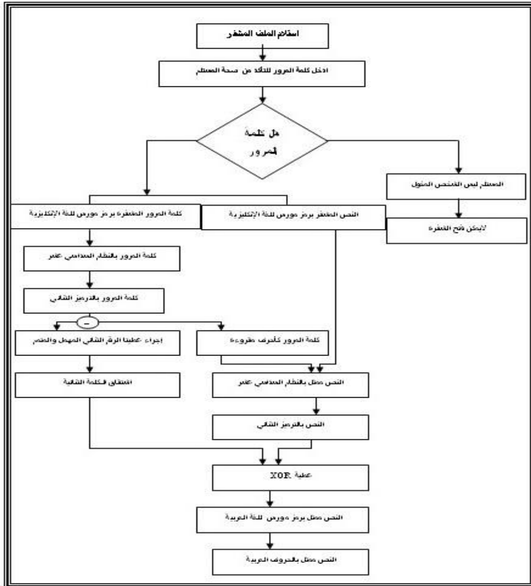
الشكل (9) خوارزمية فك الشفرة
