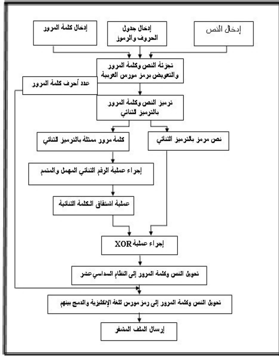
الشكل (5) خوارزمية التشفير
