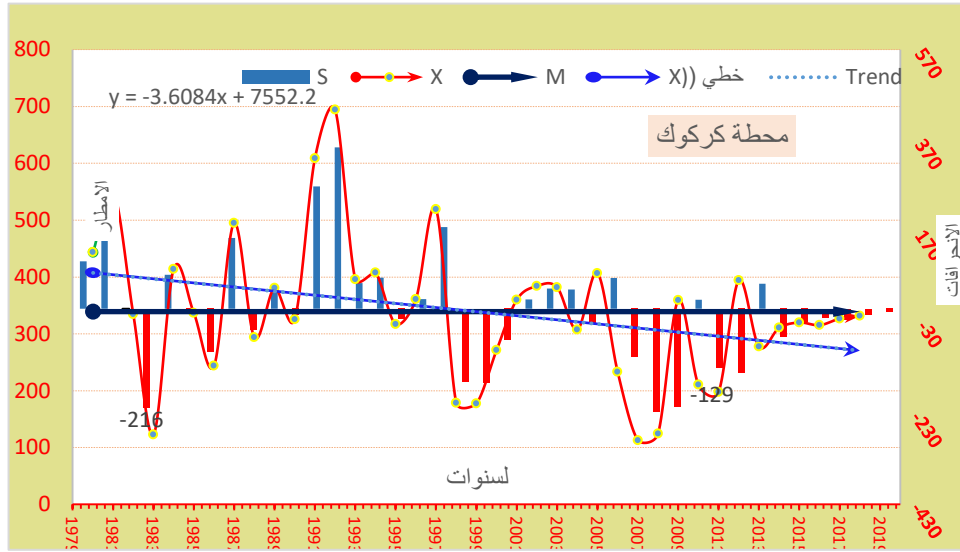
شكل (١) يبين المجاميع السنوية لأمطار محطة كركوك للمدة (١٩٨٠-٢٠١٩).
