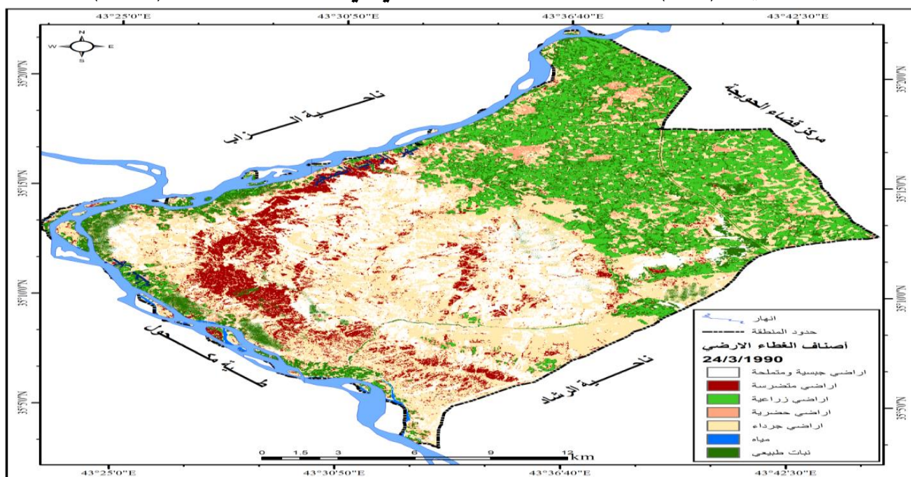
خريطة (٢-١) التصنيف الموجه للغطاء الأرضي في منطقة الدراسة لسنة (١٩٩٠)
