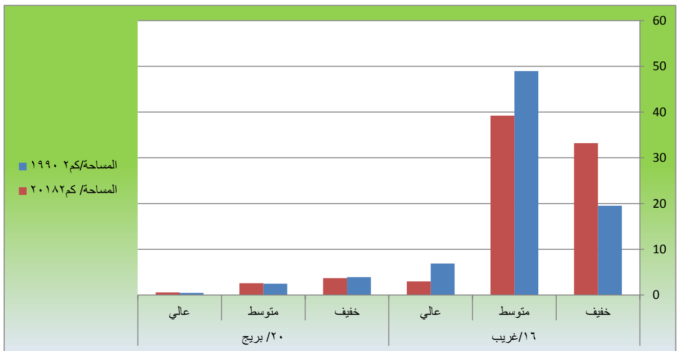
الشكل (٢-١) مساحة دليل الاخضرار (NDVI) لمنطقة الدراسة للمدة (١٩٩٠-٢٠١٨)
