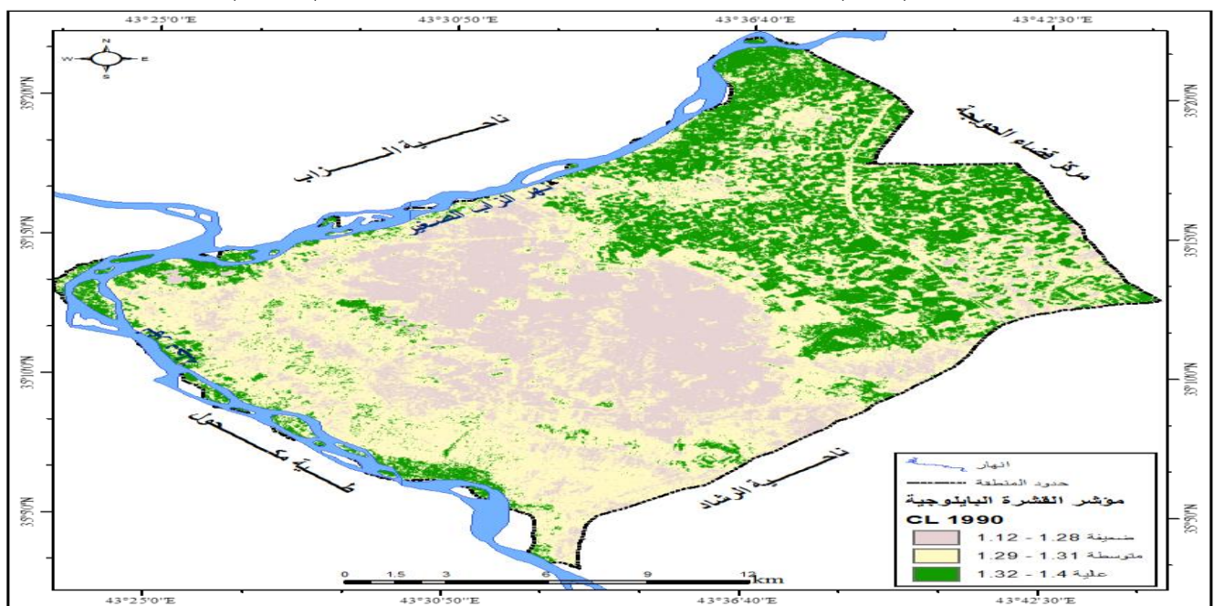
خريطة (١-٦) مؤشر القشرة البايولوجية لمنطقة الدراسة لسنة (١٩٩٠)
