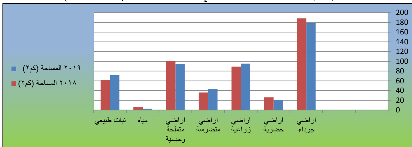
شكل (١-١) مساحة اصناف الغطاء الارضي لمنطقة الدراسة للمدة (١٩٩٠-٢٠١٨)
