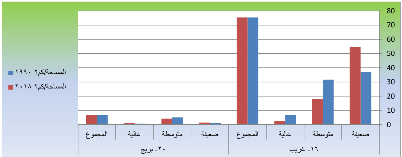
الشكل (٣-١) مساحة مؤشر دليل القشرة البايولوجية لمنطقة الدراسة للمدة (١٩٩٠-٢٠١٨)
