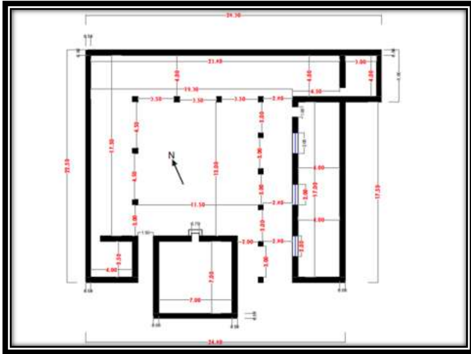
لوح (١): التخطيط الارضي لمزار محمد شرف الدين
