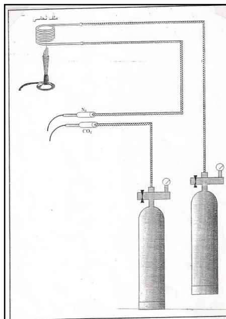
شكل (٢) جهاز الزرع اللاهوائي
