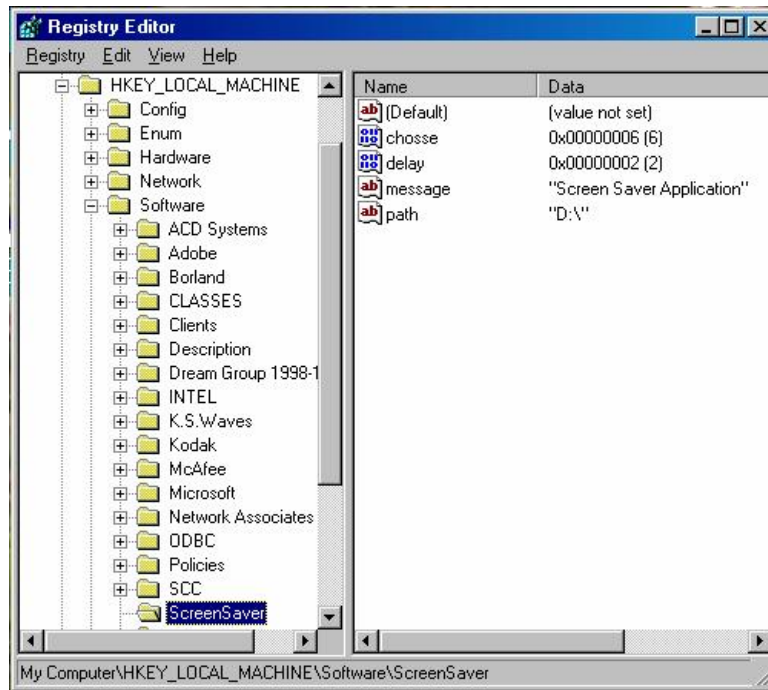
الشكل (٧) : بيانات المفتاح screensaver داخل التسجيل
