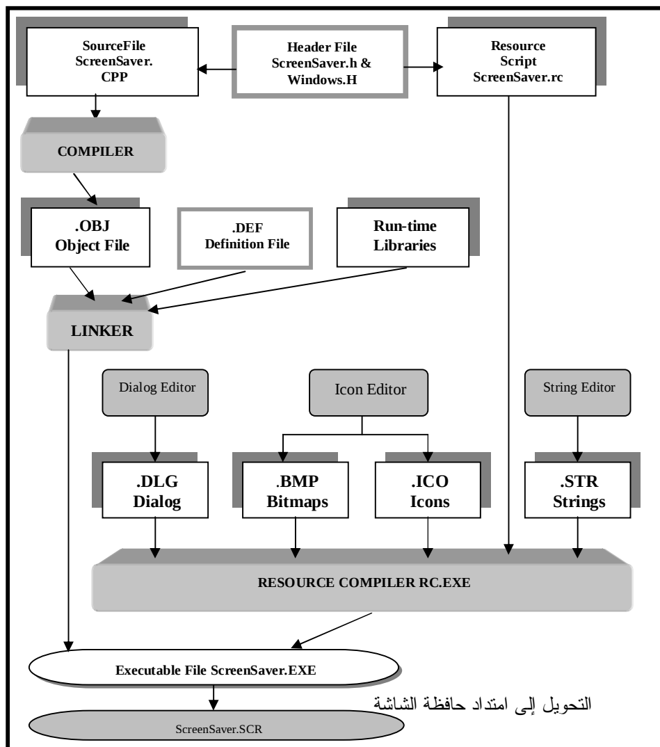
الشكل (٤) : تفاعل مكونات التطبيق مع بعضها للحصول على الملف التنفيذي
