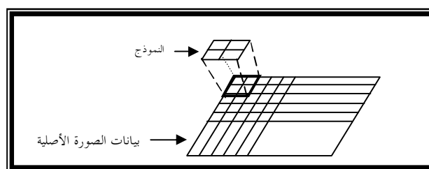
6. نزحف النموذج بمقدار وحدتين صورية إلى الأسفل (أي عمودين إلى الأسفل). الشكل (4-ب). 7. تعاد الخطوة (6-1) حتى نهاية الصورة.
