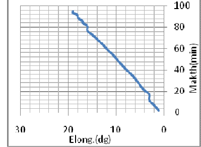
شكل(6) تغير زاوية الاستطالة مع البعد لكوكب عطارد(2\1دورة إقترانية)
