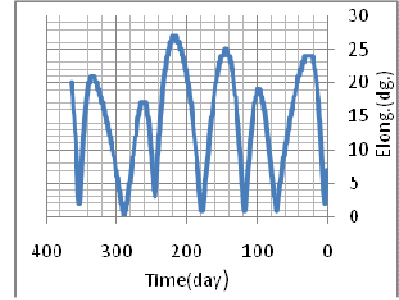
شكل(3) تغير البعد عن الارض مع الزمن لكوكب عطارد (2010)
