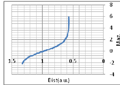
شكل(5) تغير القدر مع البعد عن الارض لعطارد(4\1دورة إقترانية)
