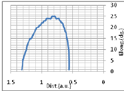
شكل(4) تغير مدة المكث مع زاوية الاستطالة لعطارد(4\1دورة إقترانية)
