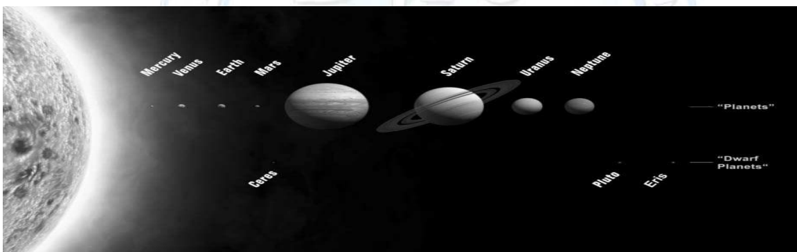
شكل (1): صورة افتراضية للكواكب السيارة [5]
