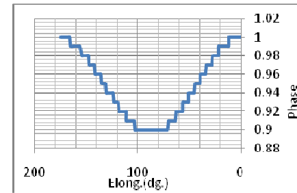
شكل(5ج) تغير القدر الظاهري مع البعد للمريخ(2\1دورة إقترانية)
