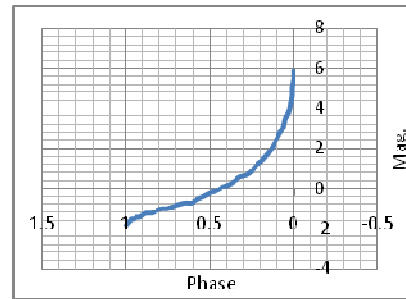
شكل(8) تغير القدر الظاهري مع الاطوار العطاردية(2\1دورة إقترانية)
