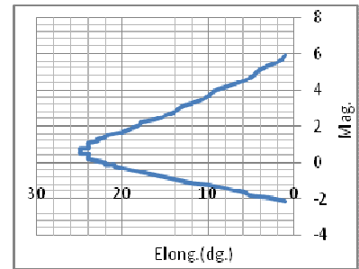
شكل(9) تغير القدر مع زاوية الاستطالة لعطارد(2\1دورة إقترانية)
