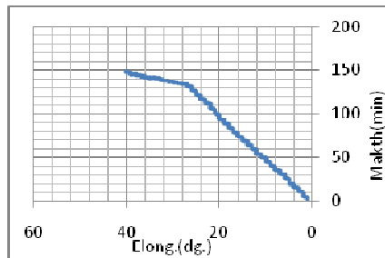
شكل(13) تغير مدة المكث مع زاوية الاستطالة للزهرة(4\1دورة إقترانية)
