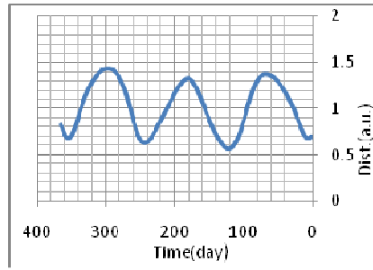
شكل(2) تغير البعد عن الارض مع الزمن لكوكب عطارد (2010)
