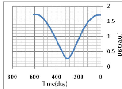
شكل(11) تغير البعد عن الارض مع الزمن للزهرة (دورة إقترانية)
