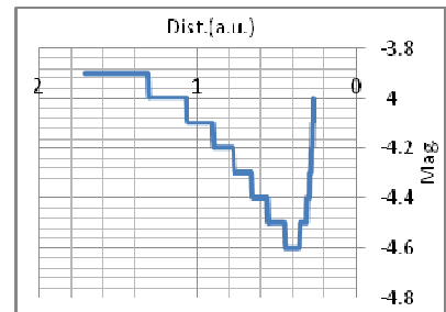
شكل(15) تغير القدر مع البعد عن الارض للزهرة(2\1دورة إقترانية)
