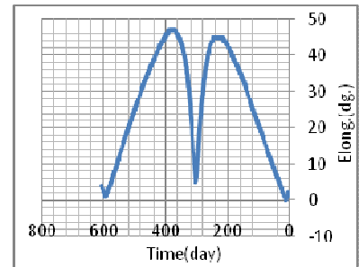
شكل(12) تغير زاوية الاستطالة مع الزمن للزهرة (دورة إقترانية)
