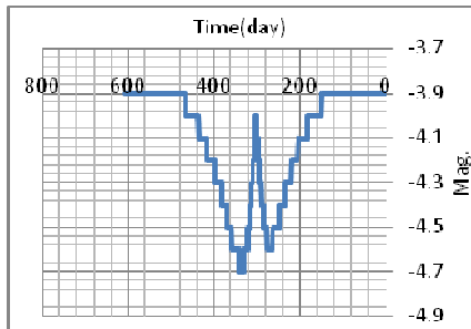
شكل(10) تغير القدر الظاهري مع الزمن للزهرة (دورة إقترانية)
