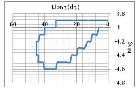
شكل(7ب) تغير الـقدر مع زاوية الاستطالة للزهرة (2\1دورة إقترانية)
