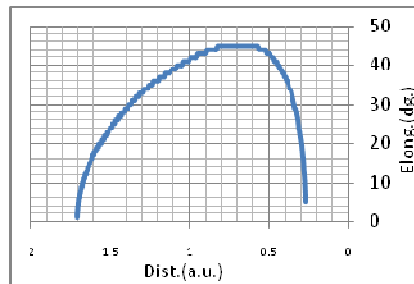
شكل(14) تغير زاوية الاستطالة مع البعد للزهرة(2\1دورة إقترانية)
