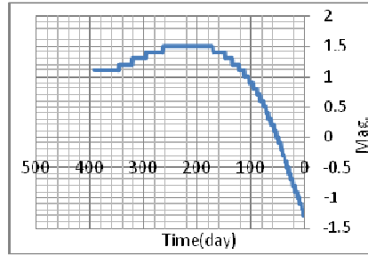
شكل(8ب) تغير القدر والاستطالة والقطر مع الزمن للزهرة (دورة إقترانية) شكل(1ج)تغير زاوية الاستطالة مع الزمن للمريخ (2\1دورة إقترانية)
