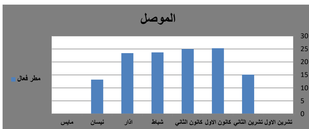
الشكل (١٠) نتائج قيم المطر الفعّال (ملم) للمدة (1988-2018) لمحطة الموصل
