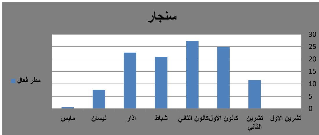
الشكل (١٣) نتائج قيم المطر الفعّال (ملم) للمدة (1988-2018) لمحطة سنجار
