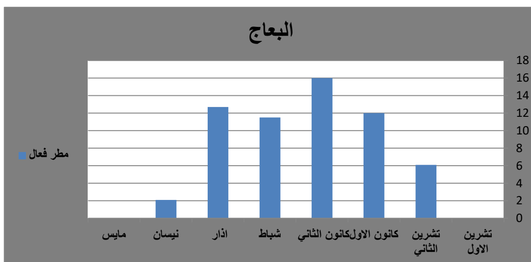
الشكل (١٤) نتائج قيم المطر الفعّال (ملم) للمدة (1988-2018) لمحطة البعاج
