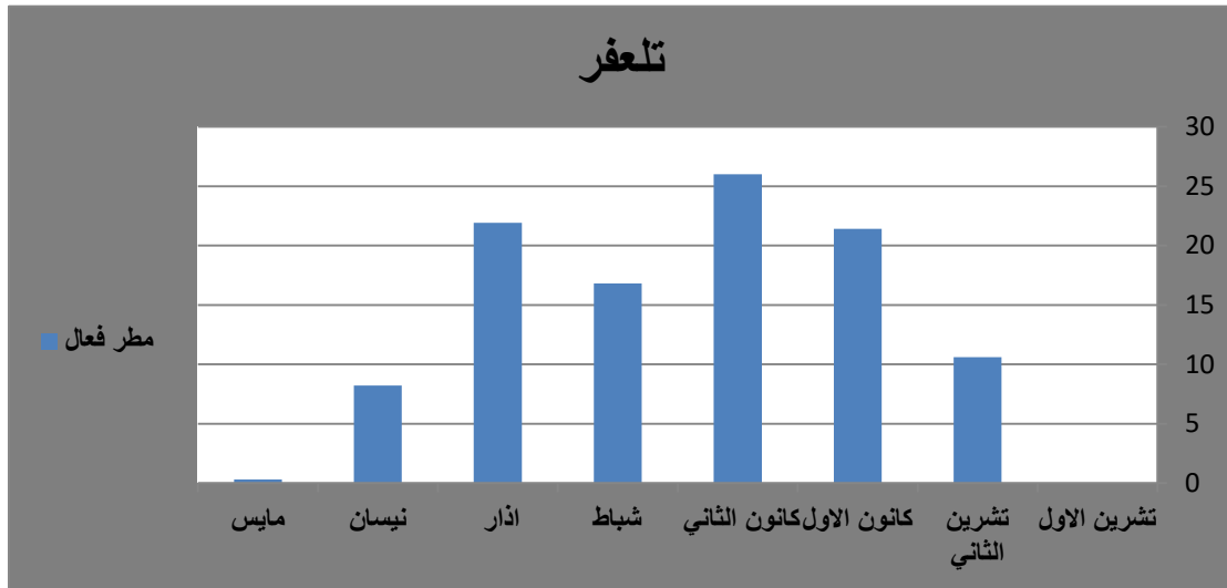
الشكل (١٢) نتائج قيم المطر الفعّال (ملم) للمدة (1988-2018) لمحطة تلعفر
