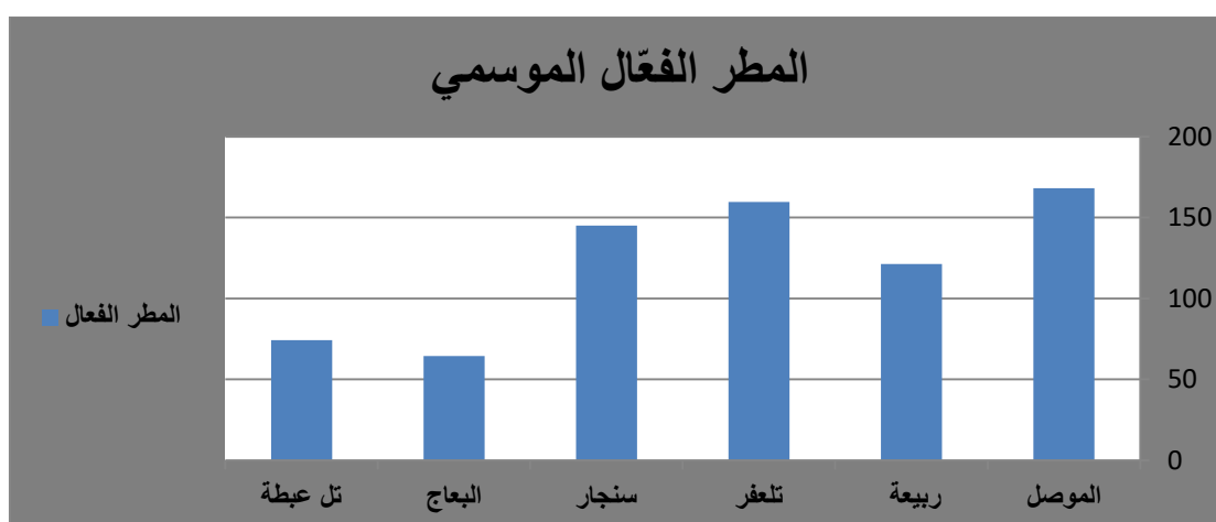
الشكل (٢) مجموع المطر الفعّال (ملم) السنوي لمحطات منطقة الدراسة للموسم المطري (1989-1990)
