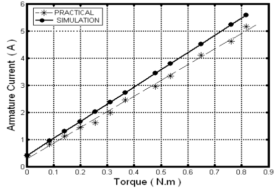
الشكل (٦) مقارنة نتائج العزم مع تيار المنتج
