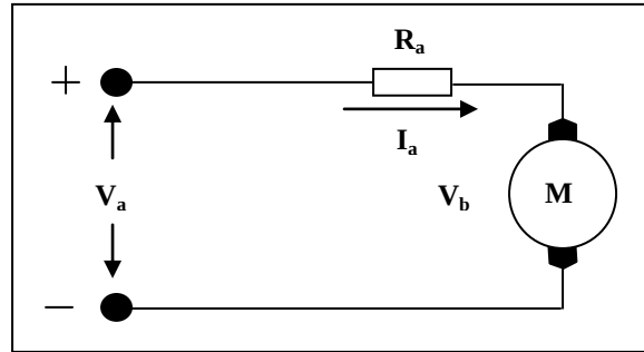
الشكل (٢) الدائرة المكافئة لمحرك المغناطيس الدائم المثالي في حالة اللاحمل .
