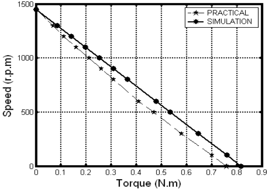
الشكل (٧) مقارنة نتائج العزم مع السرعة
