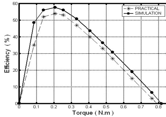
الشكل (٨) مقارنة نتائج العزم مع الكفاءة
