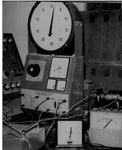
الشكل ( ٥ ) صورة توضح اختبار التحميل للمحرك .
