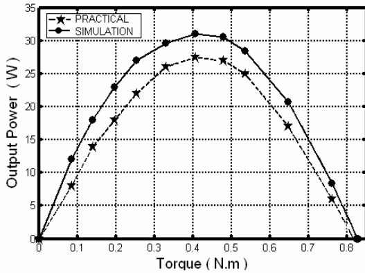
الشكل (٩) مقارنة نتائج العزم مع القدرة الخارجة
