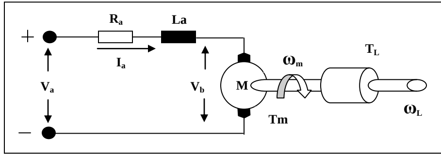
الشكل ( ٣ ) الدائرة المكافئة لمحرك (PMDCM) في حالة الحمل .
