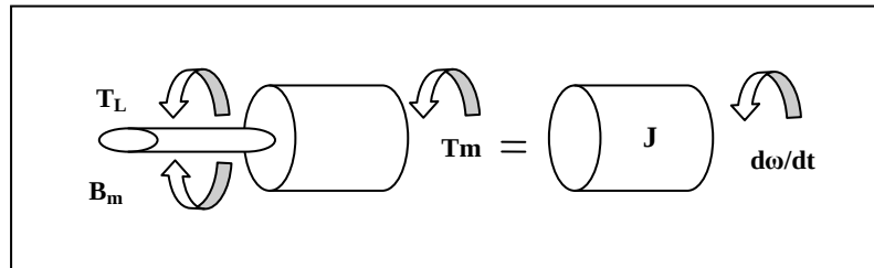
الشكل ( ٤ ) مخطط حركي للجسم الحر لدوار المحرك .
