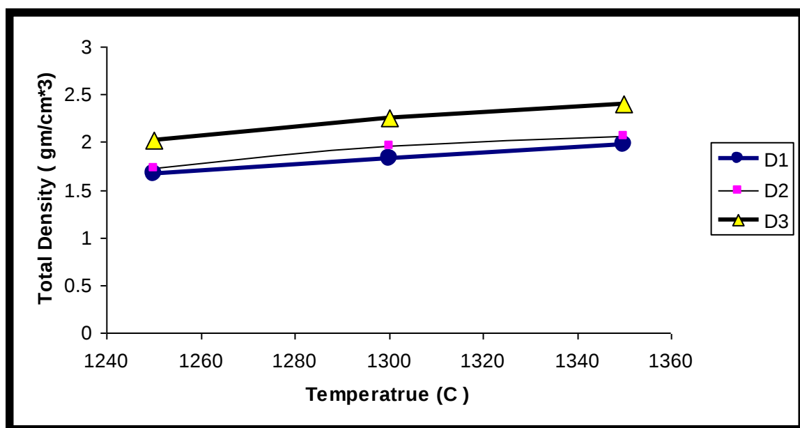
شكل (2) يوضح العلاقة بين الكثافة الإجمالية ( \text{gm/cm}^3 ) دالة لدرجة حرارة الحرق للمجاميع السيراميكية D1,D2,D3
