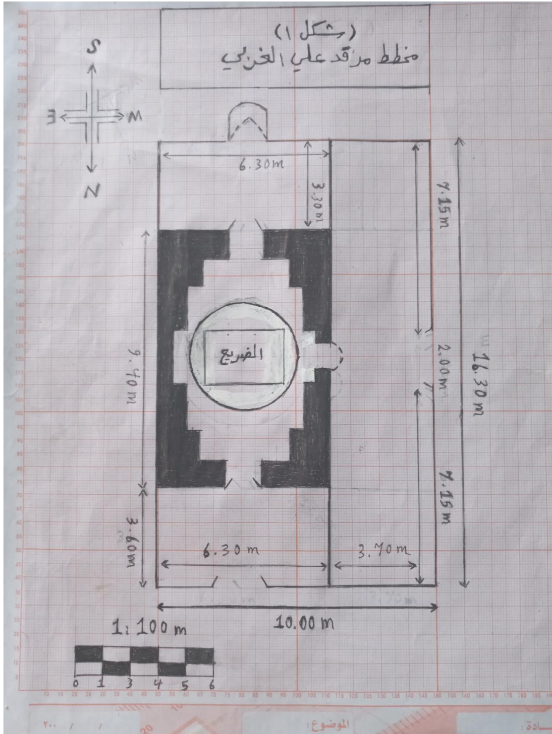
(شكل ١) مخطط مرقد علي الغربي المصدر : الهيئة العامة للمساحة -
