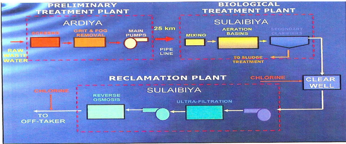
شكل رقم (٢) مراحل معالجة المياه الداخلة في محطة الصليبية -الاولية - والبيولوجية-والتطهير
