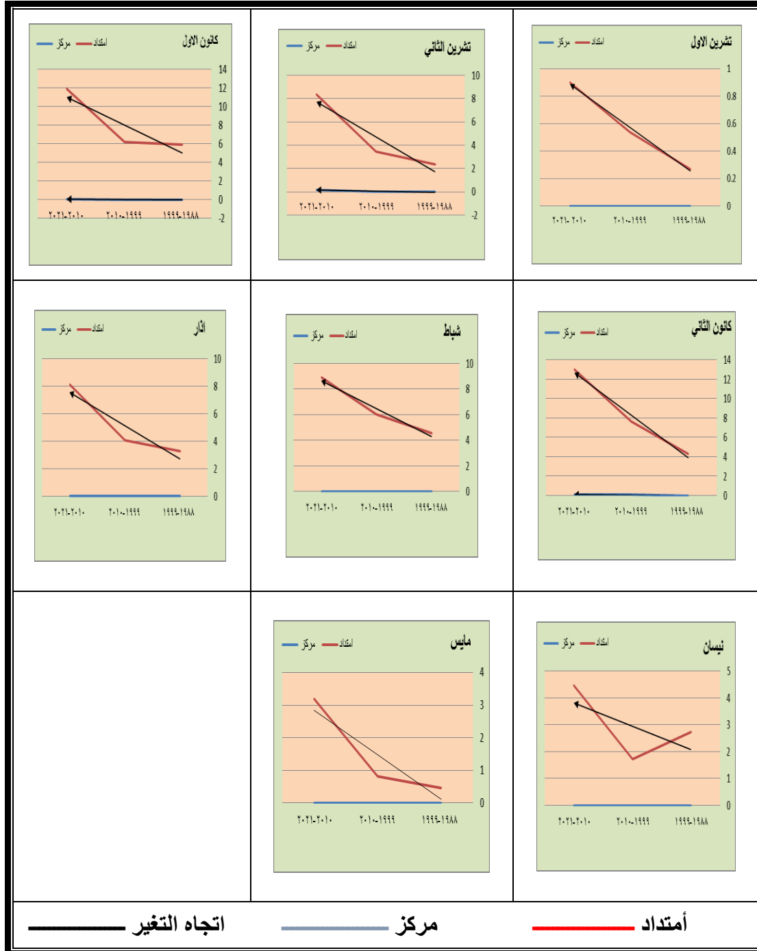
شكل (٢) معدل عدد ايام بقاء المرتفع السيبيري (يوم) ومقدار تغيرها فوق محافظة البصرة الرصد (GMT12) للدورة الثانية (١٩٨٨-٢٠٢١)
