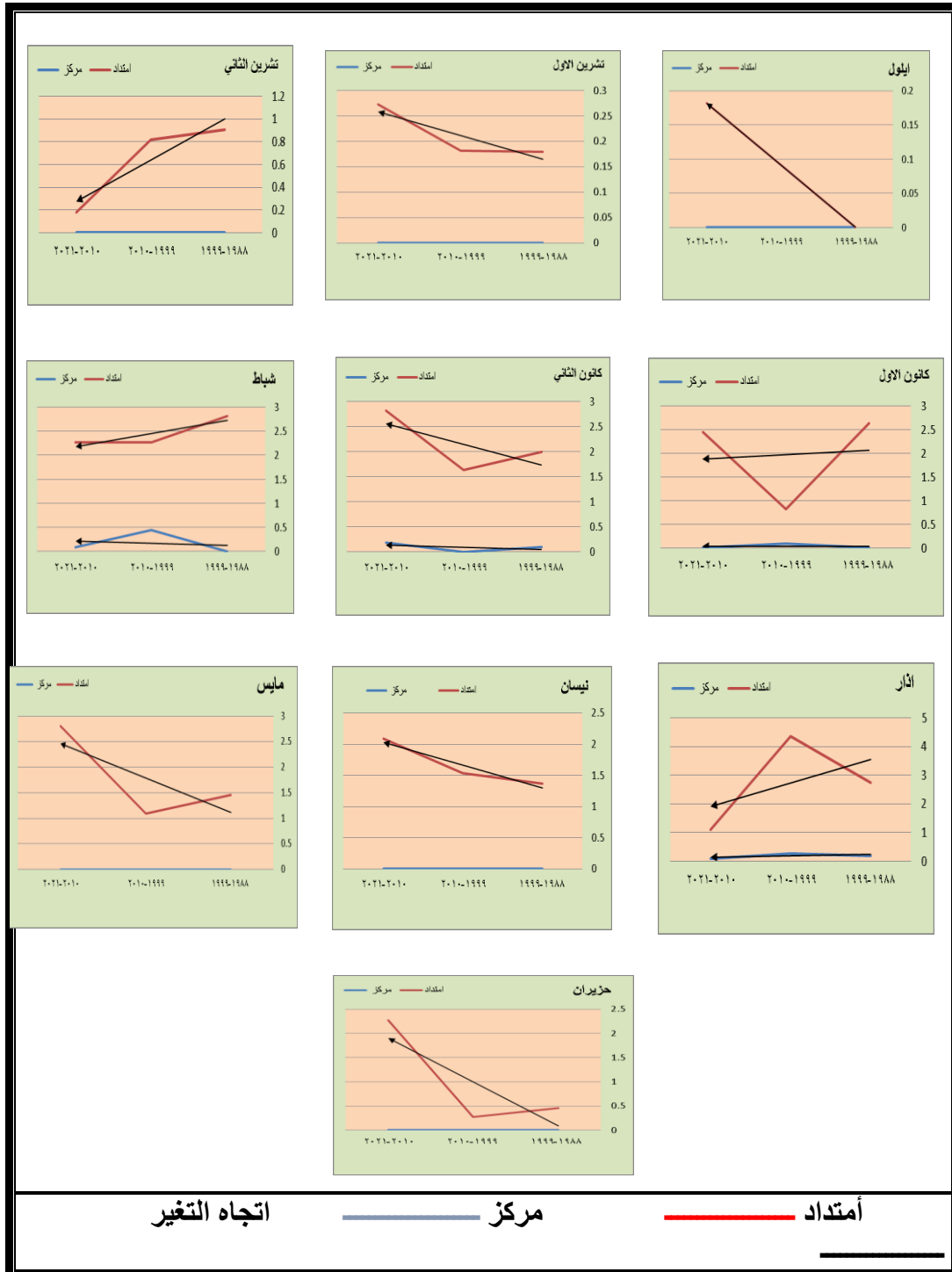
شكل (٦) معدل عدد ايام بقاء المرتفع الشبه المداري (يوم) واتجاه تغيره فوق محافظة البصرة للدورة الثانية (١٩٨٨-٢٠٢١) للرصدية (GMT12z)
