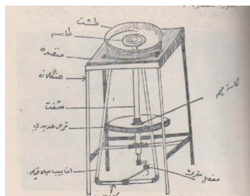
شكل رقم ١٦ (مخطط دولاب لصنع الفخار)
