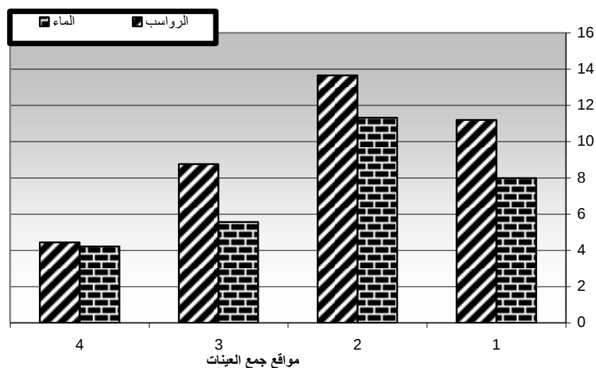
الشكل ( 3 ) تركيز عنصر الرصاص في المياه ( مليغرام/لتر ) والرواسب ( مليغرام / غم ) في مواقع جمع العينات على نهر شط العرب
