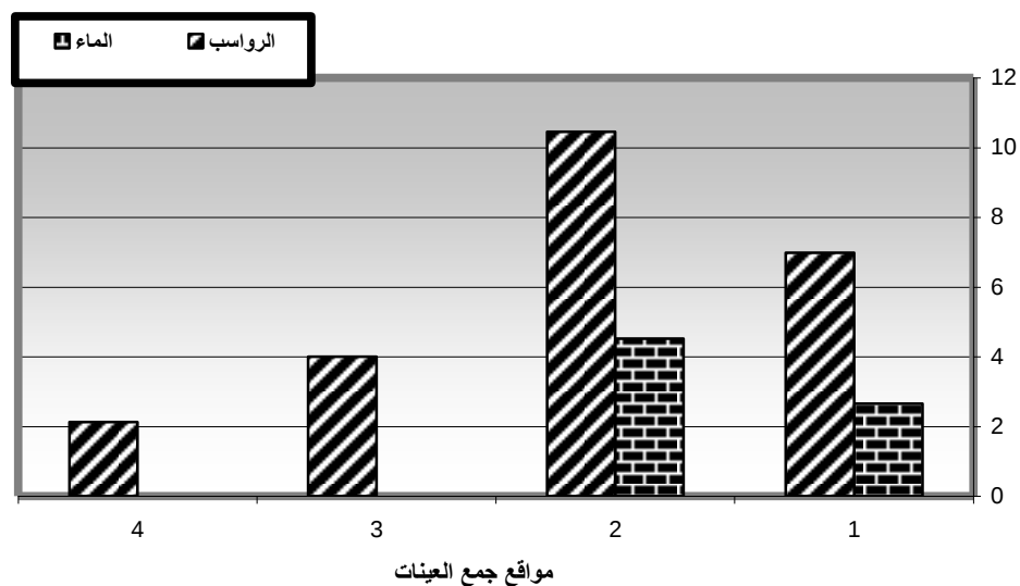
الشكل ( 2 ) تركيز عنصر النحاس في المياه (مليغرام/ لتر ) والرواسب ( مليغرام/ غم ) في مواقع جمع العينات على نهر شط العرب
