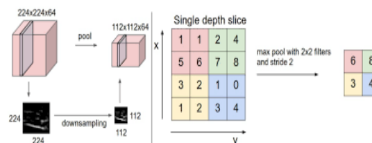
Fig. 3. Pooling Layer.
