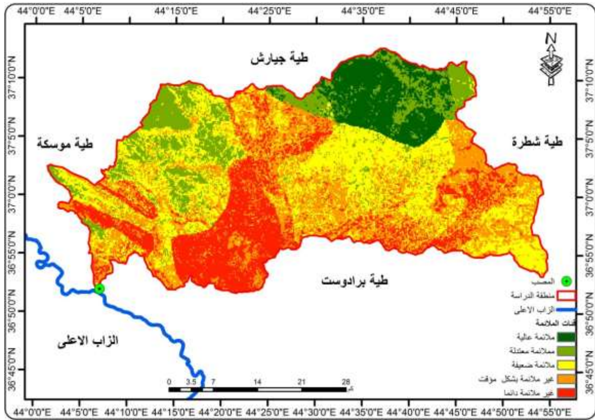
خريطة (٣) الملائمة الأرضية في حوض وادي ريزان
