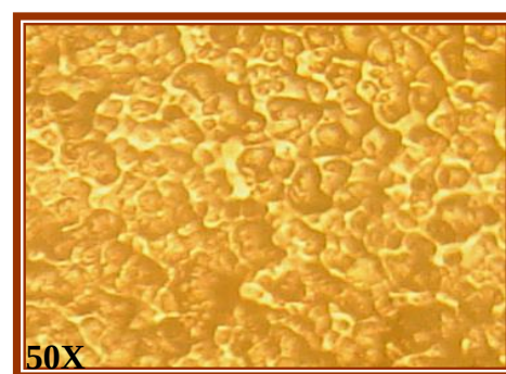
10% Al 2 O 3
