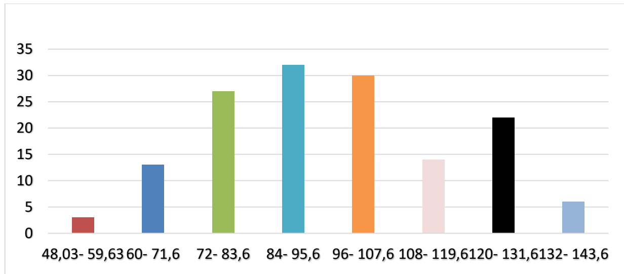
شكل (١) المدرج التكراري لسرعة المركبات في منطقة الدراسة
