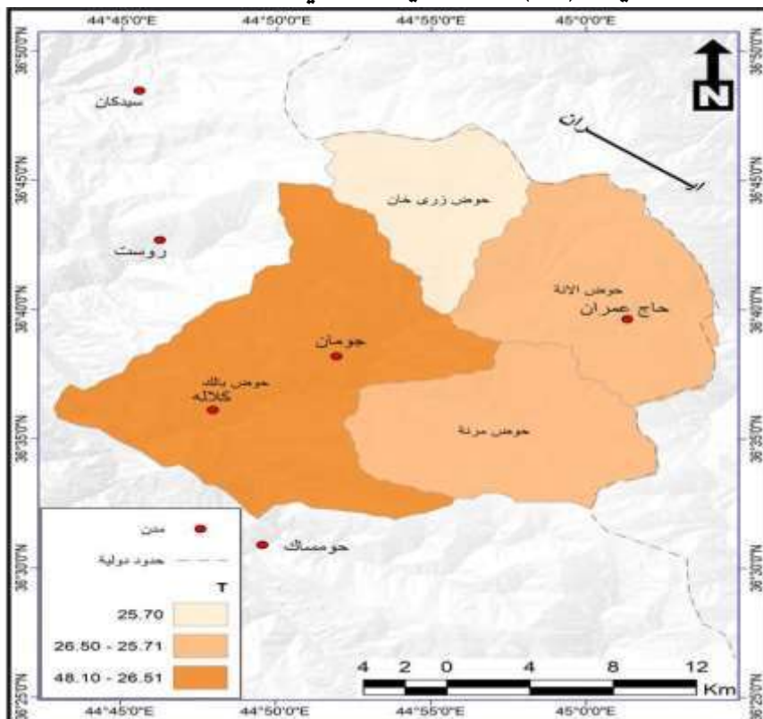
خريطة (11) مدة الجريان السيلي لأحواض منطقة الدراسة
