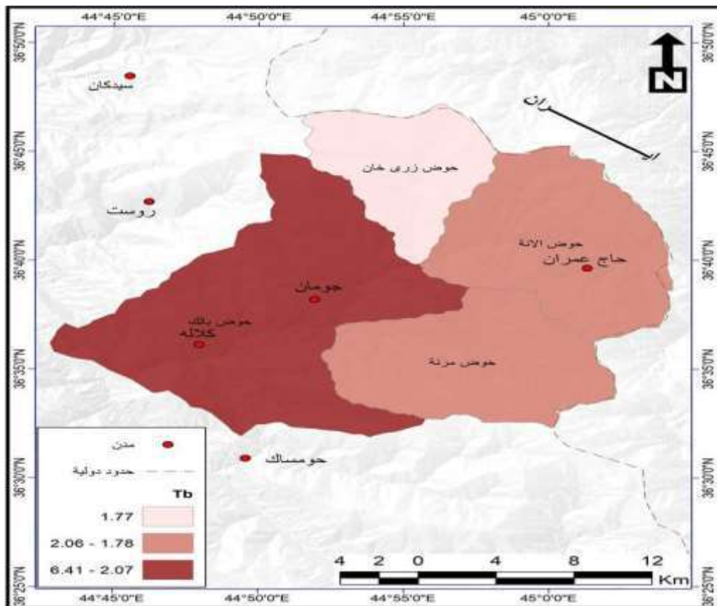
خريطة (8) زمن الاساس للسيول (Tb day) لأحواض منطقة الدراسة
