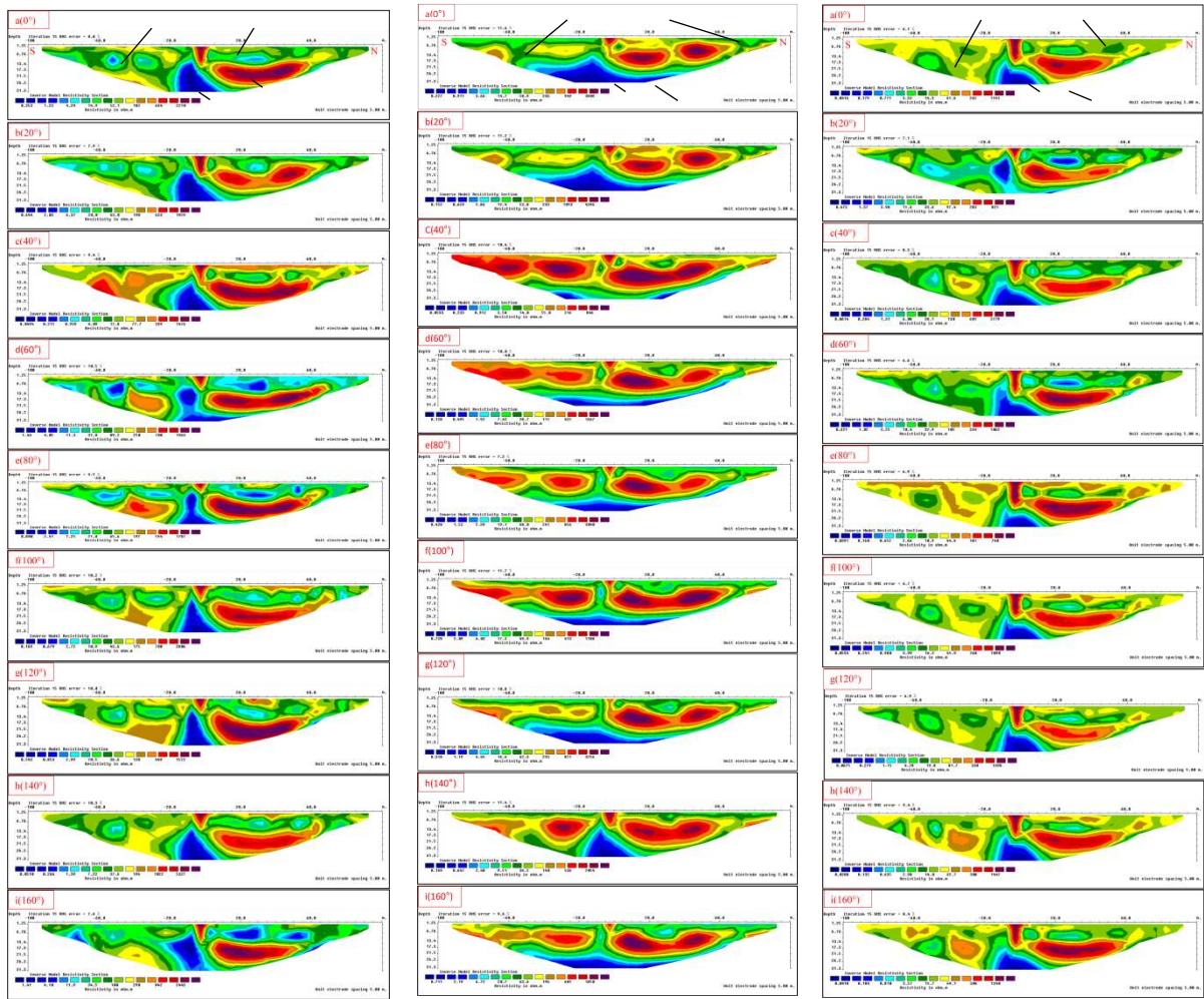
الشكل 11: موديلات المقاومة المعكوسة لمقاطع التصوير الاتجاهي في S-4.
