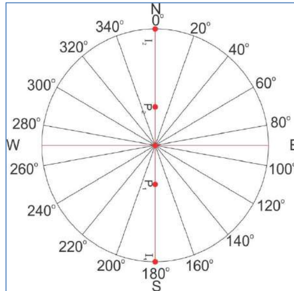
الشكل 2: النمط الهندسي لمقاطع التصوير المقاومي الكهربائي الاتجاهي (Azimuthal 2D Resistivity Imaging) في مواقع الدراسة الحالية.
