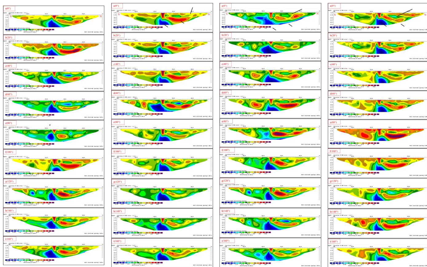
الشكل 15: موديلات المقاومة المعكوسة لمقاطع التصوير الاتجاهي في >S-8
