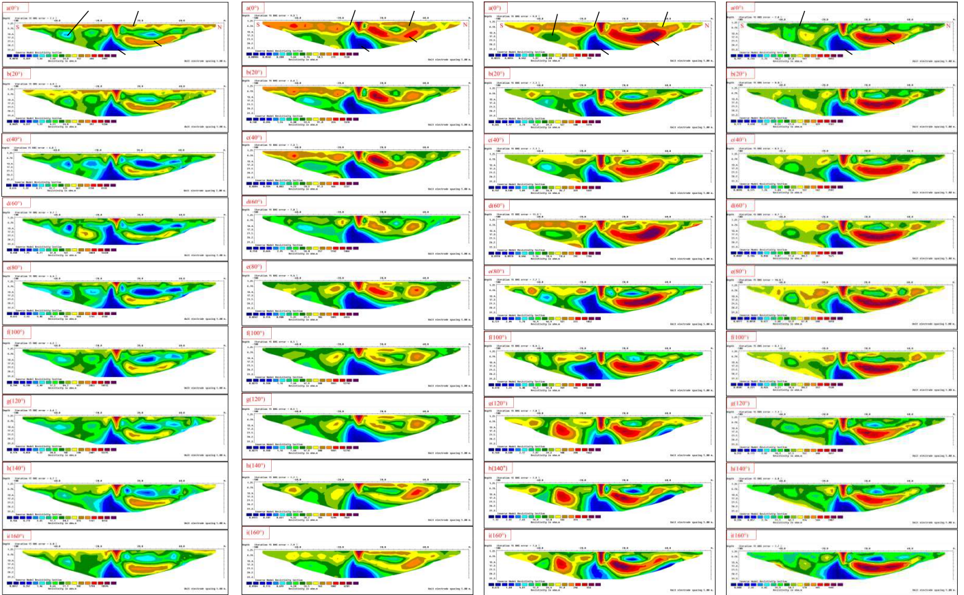
الشكل 6: موديلات المقاومة المعكوسة لمقاطع التصوير الاتجاهي في S-7.
