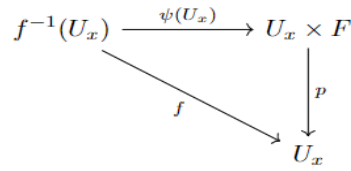
Fig. 1. : Fiber bundle
