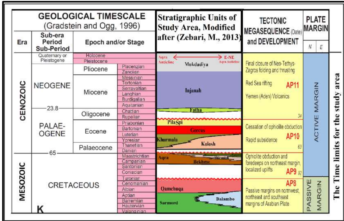
الشكل 4: التتابعات الطباقية التكتونية الكبيرة (TMS) لمنطقة الدراسة، معدل عن (Sharland et al., 2001).
