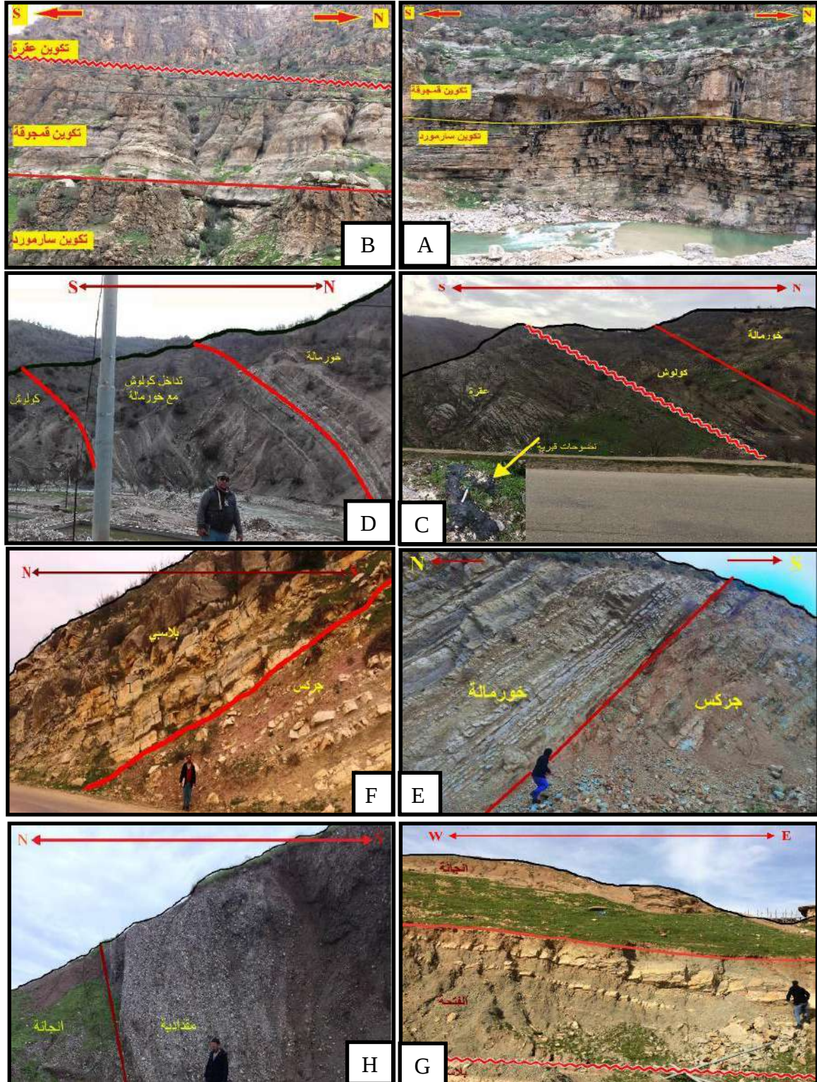
اللوحة 1: توضيح صور حقلية للتكوينات المنكشفة في طية عقرة المحدبة مع طبيعة حدود التماس فيما بينها.
