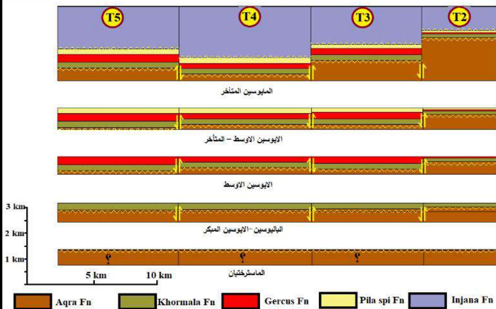
الشكل 9: موديل يوضح الحركة العمودية للفوالق المستعرضة وتأثيراتها على التغير الجانبي لسمك التكاوين في طية عقرة المحدبة.
