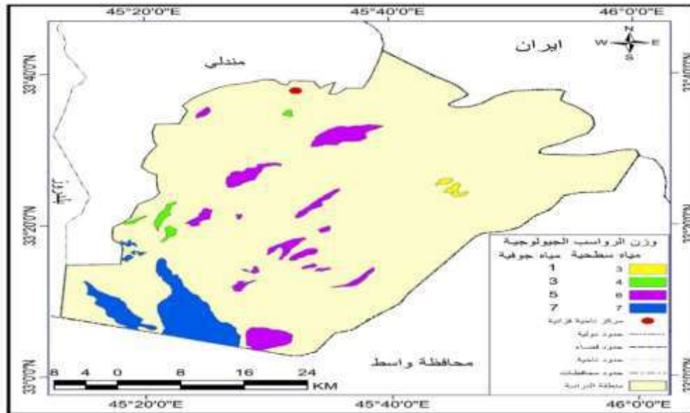
الخريطة (6) اوزان المنخفضات حسب التكوينات والرواسب الجيولوجية في منطقة الدراسة
