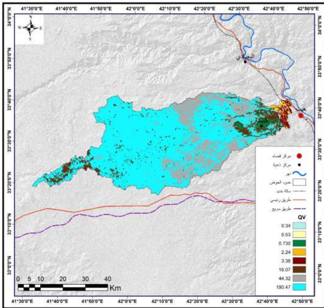
خريطة (١٠) حجم الجريان السطحي Qv في المنطقة
