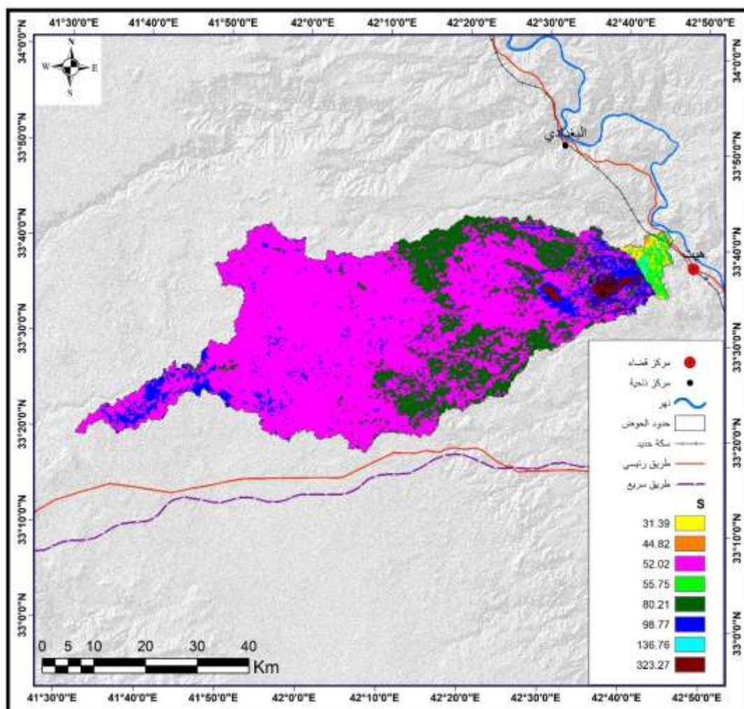
خريطة (٧) توزيع فئات قيم معامل (S) في المنطقة
