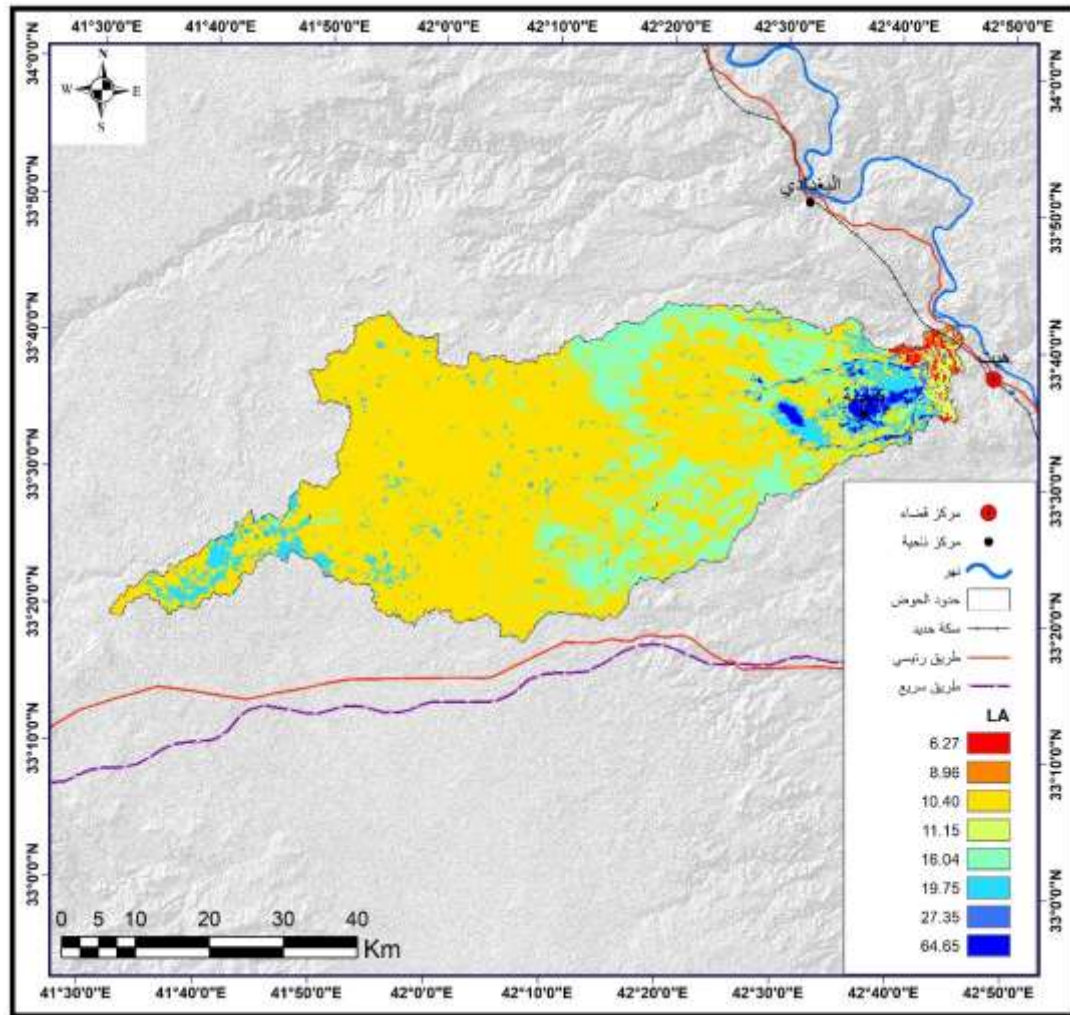
خريطة (٨) فئات قيم معامل الاستخلاص الاول (la) في المنطقة
