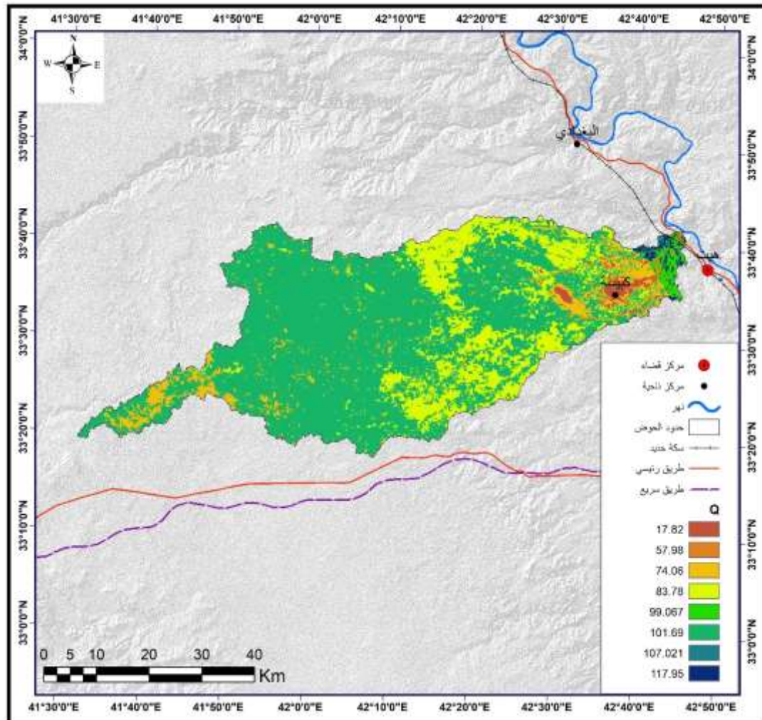
خريطة (٩) فئات قيم معامل (Q) في المنطقة
