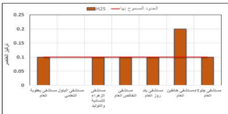
شكل (3) نسبة غاز H 2 S المنبعث من محارق مستشفيات منطقة الدراسة
