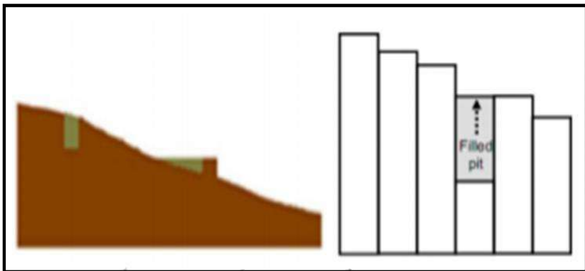
صورة 3: توضيح معالجة القيم الشاذة بالارتفاع أو الانخفاض.
