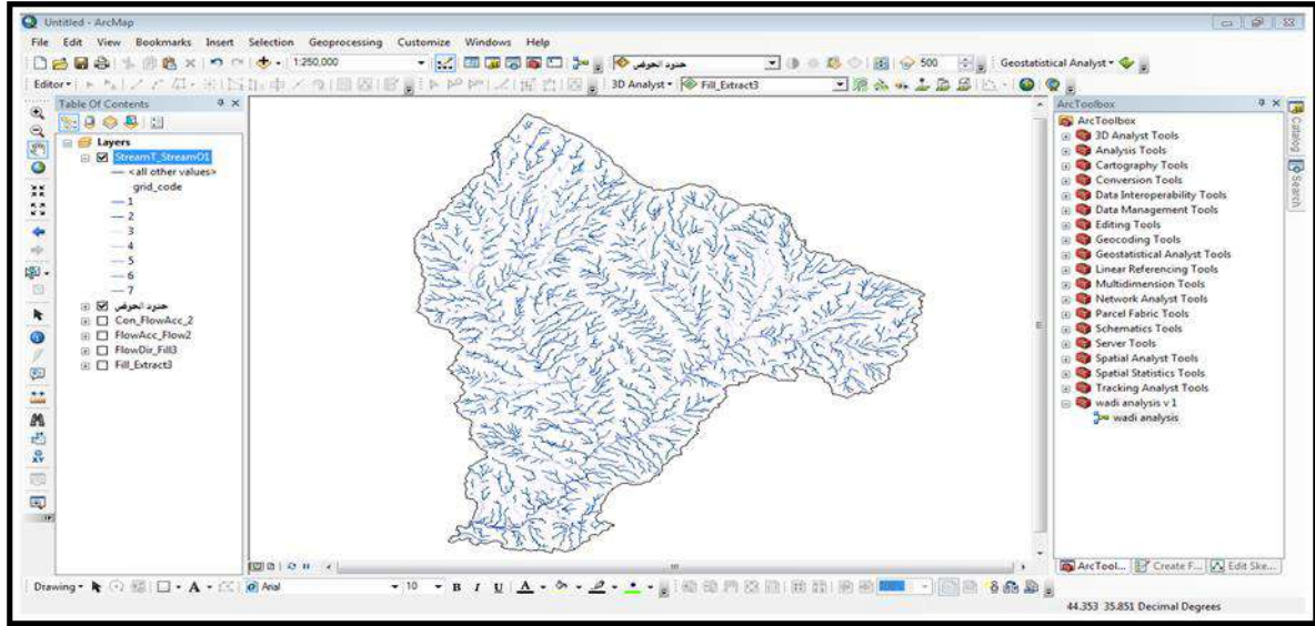
صورة 8: توضيح الرتب النهرية في الحوض.
