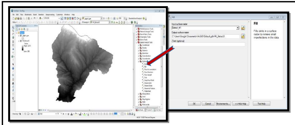
صورة 4: توضح كيفية استخدام الامر (Fill) لمعالجة القيم الشاذة.
