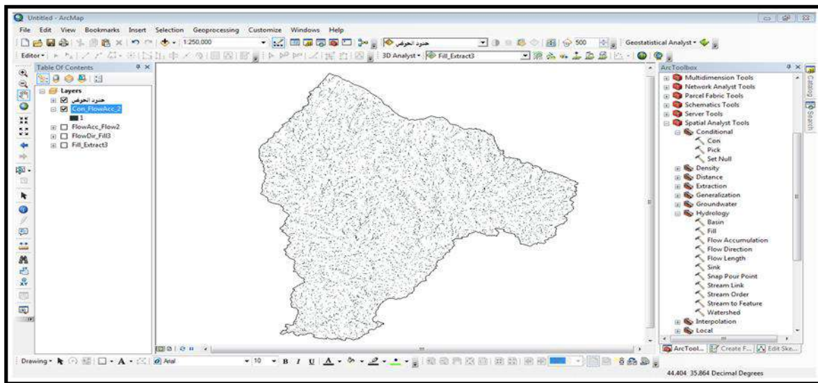
صورة 7: توضح المجاري الفرعية في الحوض.
