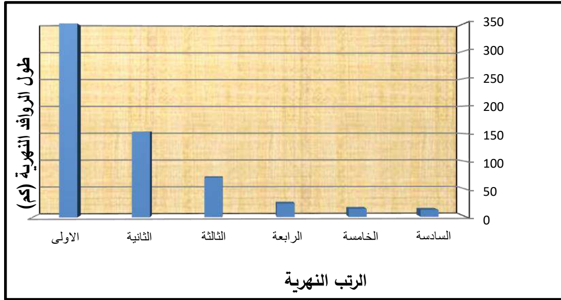
الشكل 7: العلاقة بين الرتب النهرية واطوالها.
