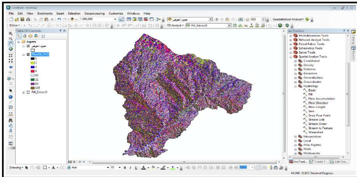
صورة 5: توضح اتجاهات الجريان في الحوض.
