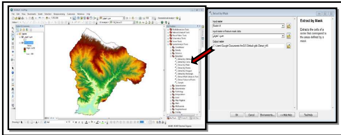
صورة 2: توضيح كيفية استقطاع نموذج الارتفاع الرقمي (DEM) لمنطقة الدراسة.
