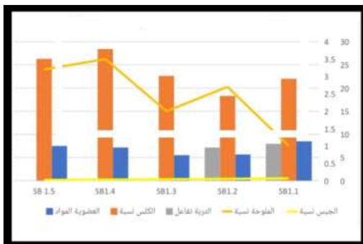
شكل رقم (٢) تربة احواض الانهار المظمورة
