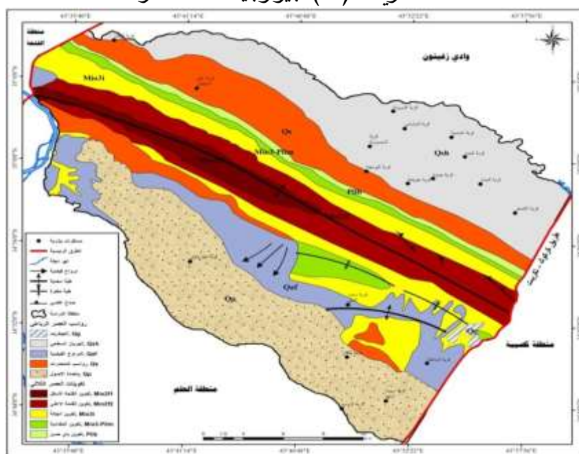
خريطة ( ٢ ) جيولوجية منطقة الدراسة
