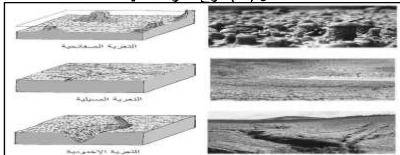
شكل ( ٢ ) انواع التعرية المائية
