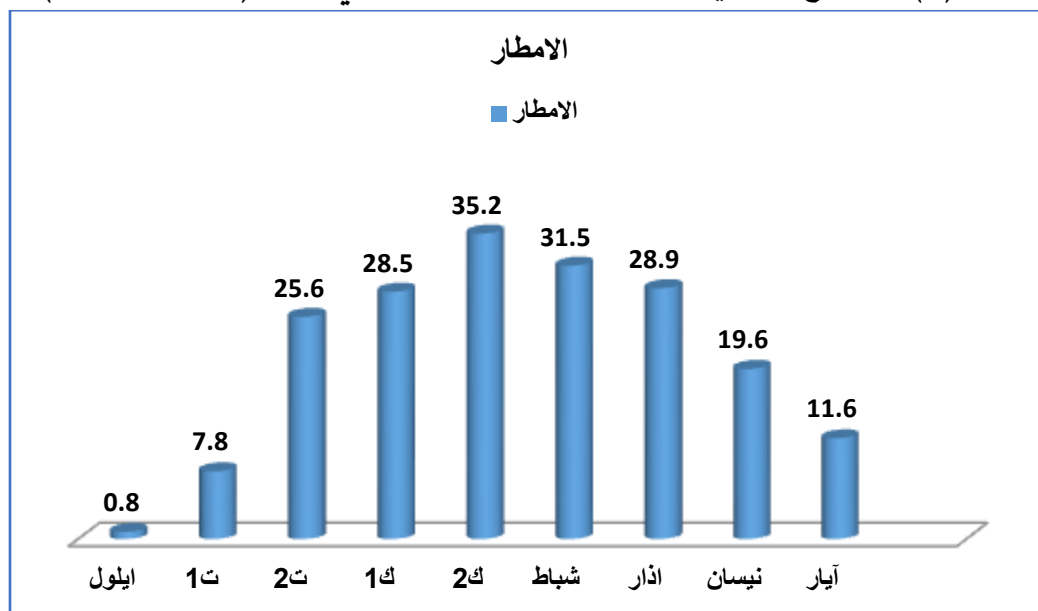
شكل (١) المجموع السنوي للأمطار الساقطة لمحطة بيجي للمدة (١٩٩١-٢٠٢٢)
