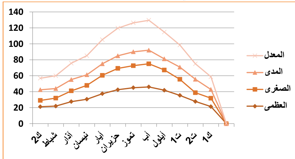
شكل (٢) المعدلات الشهرية والسنوية لدرجات الحرارة العظمى - والصغرى - والمدى - والمعدل الحراري لمحطة بيجي للمدة من (١٩٩١-٢٠٢٢)
