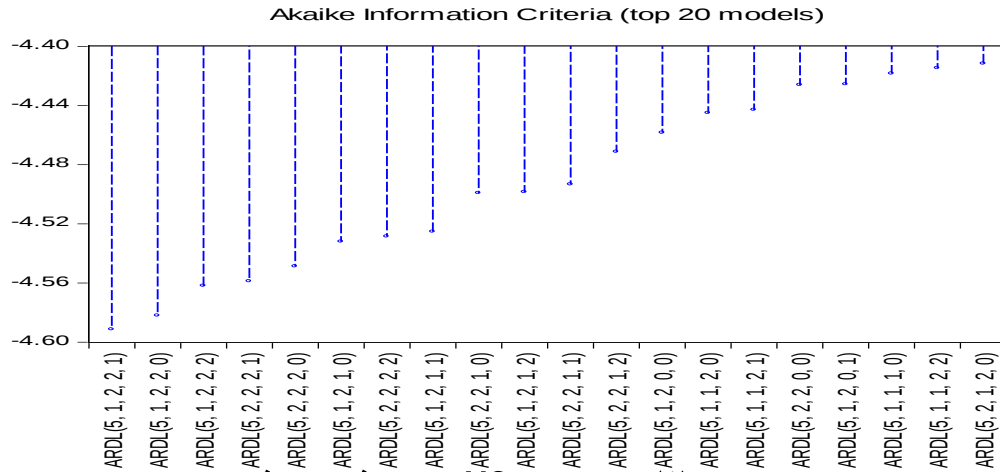
الشكل (1) نتائج اختبار AIC لتحديد افضل نموذج
